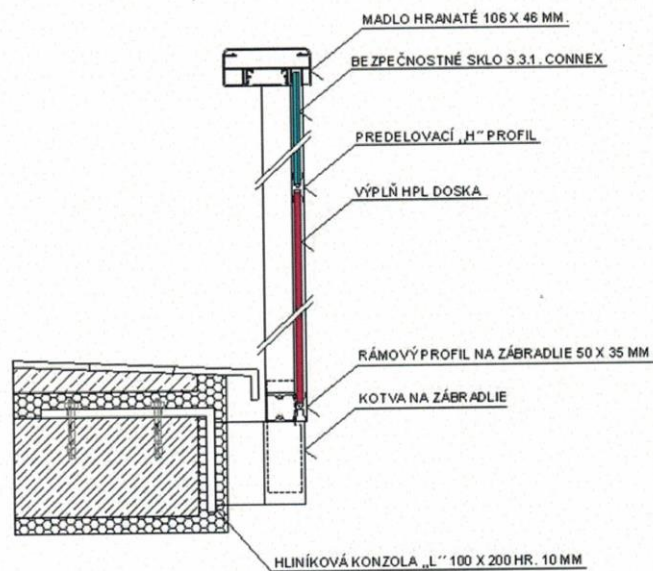
Obrázok 1 – GARO MAX GLASS (rez)
