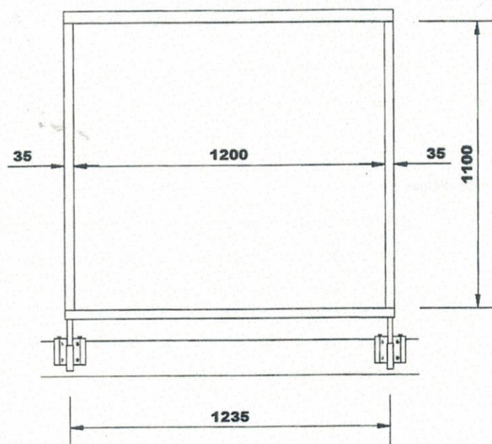
Obrázok 1 – GARO MAX GLASS (rez)
